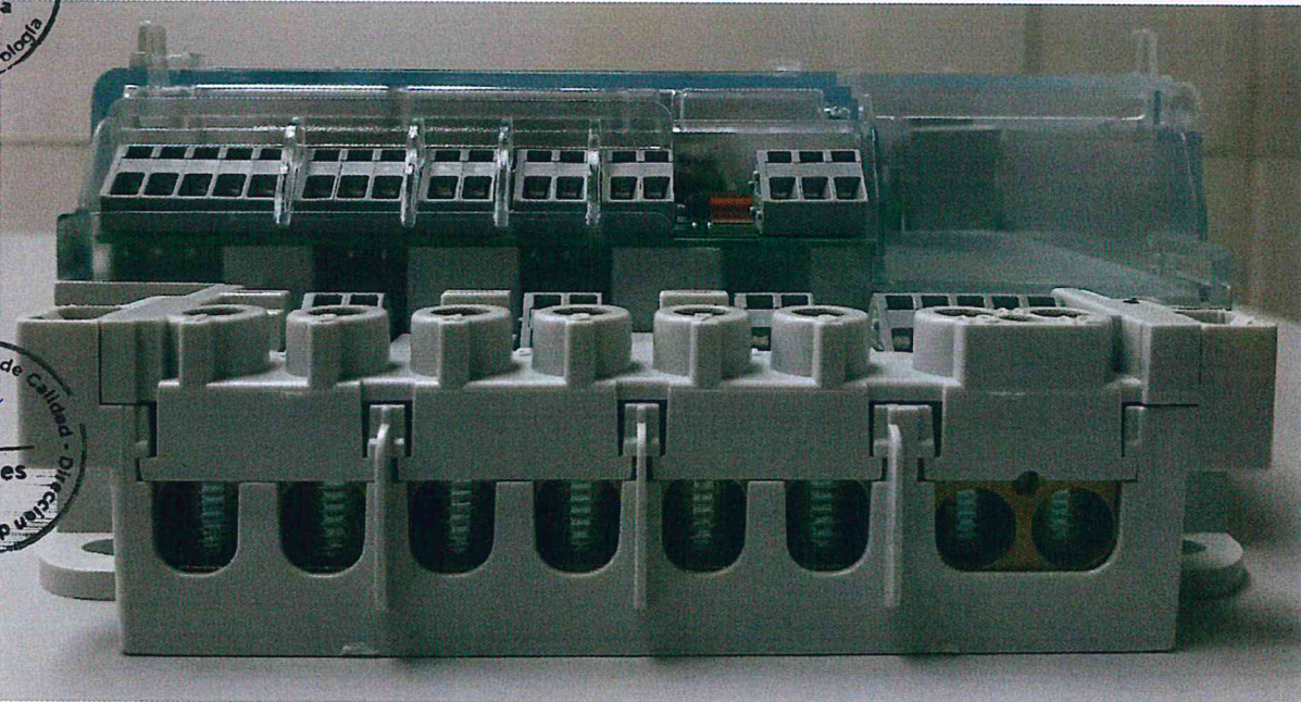
Fotografía 5. Vista inferior de los bornes del medidor evaluado
