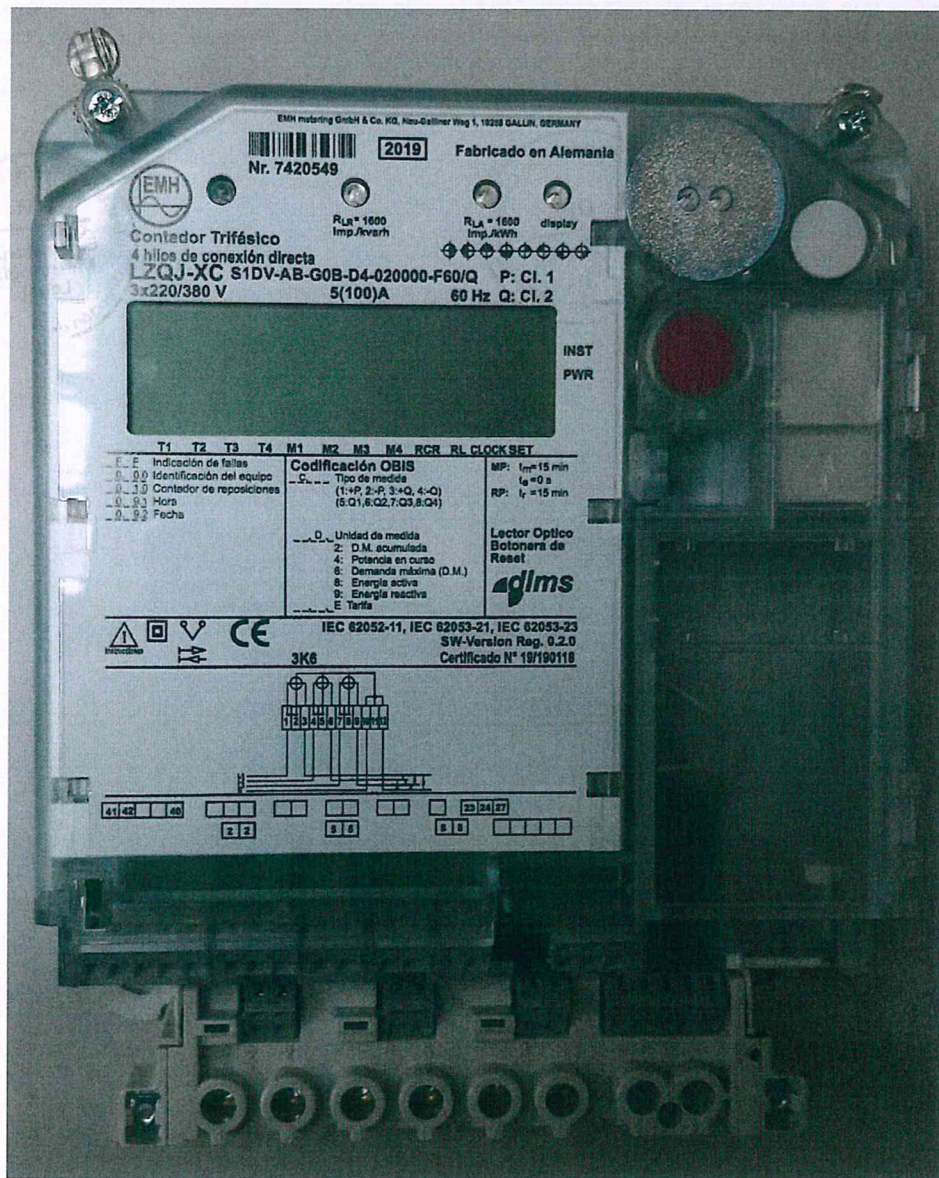
Fotografía 1. Vista frontal del medidor evaluado
