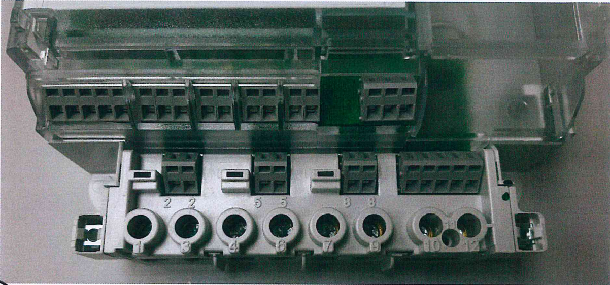
Fotografía 4. Vista superior de los bornes del medidor evaluado
