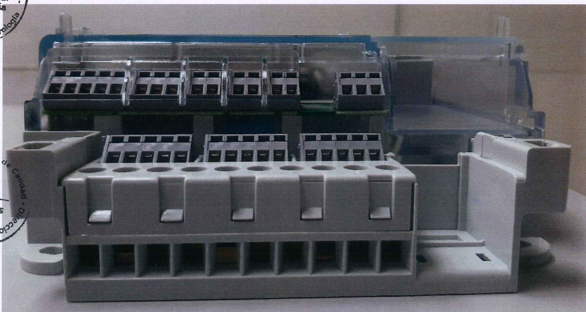
Fotografía 5. Vista inferior de los bornes del medidor evaluado
